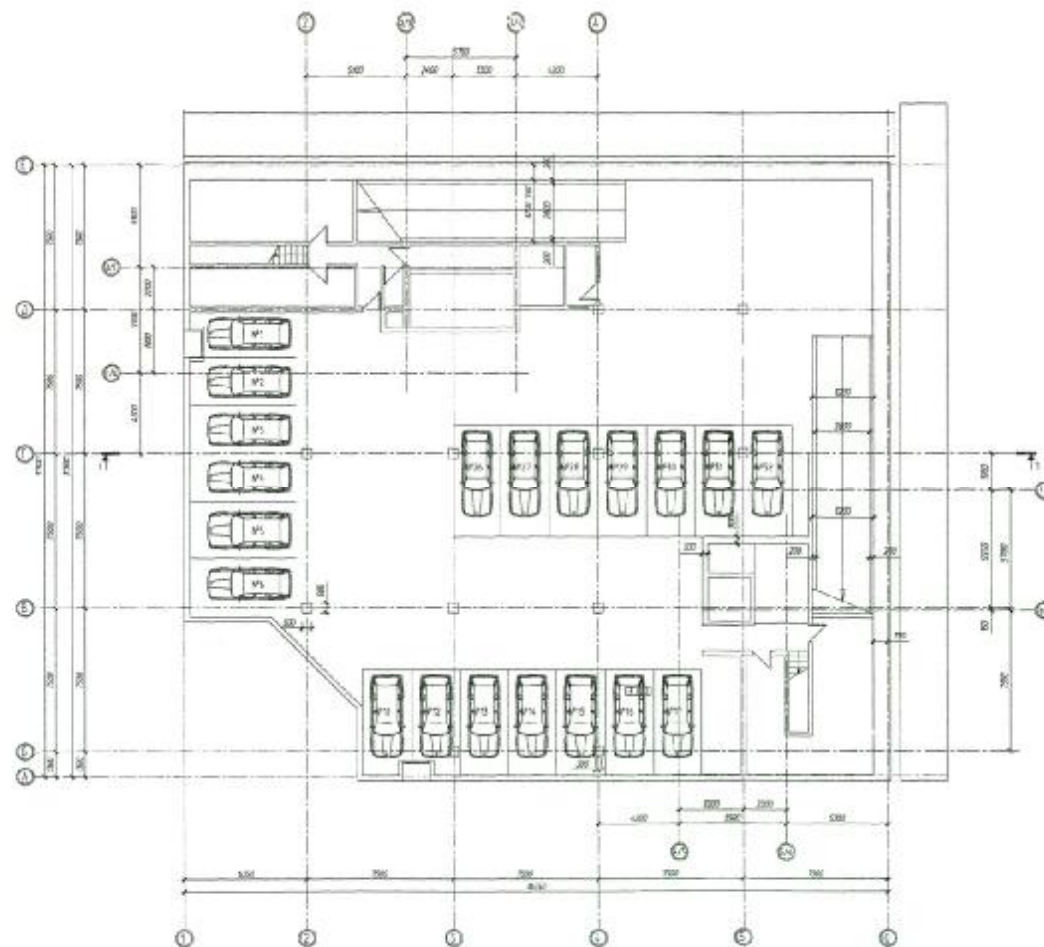
План подземного паркинга
